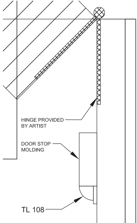
3 MOLDING DTL SCALE: 6" = 1'-0"
