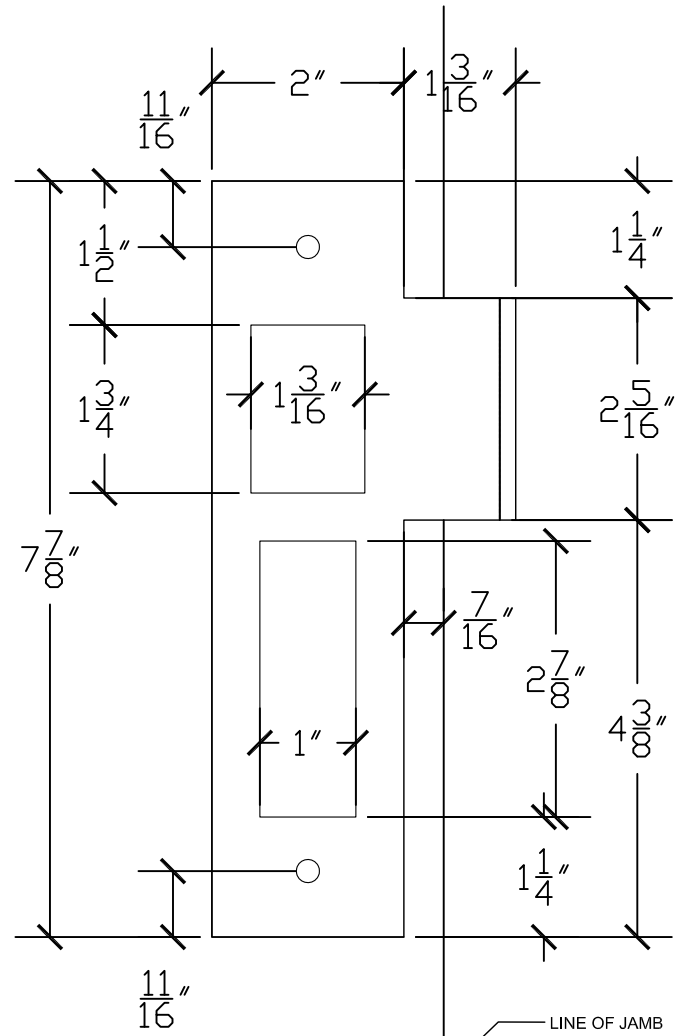
1 ELEVATION 3 SCALE: 6" = 1'-0"
